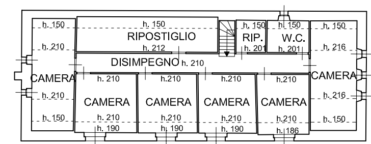
PIANTA PIANO SECONDO (SOTTOTETTO)
